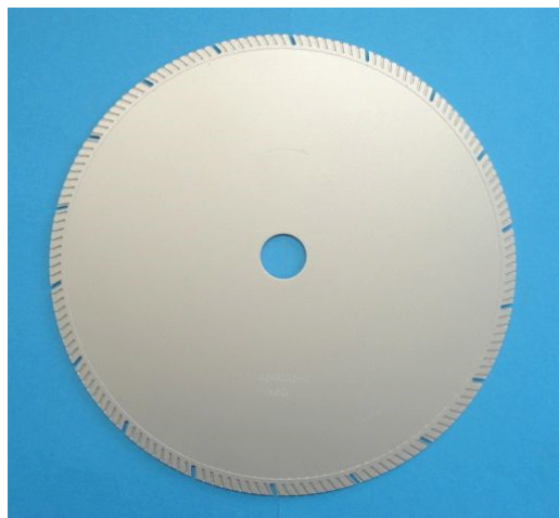
タイル用ダイヤモンドブレード 粒度#80 ・Φ260x2Tx7Wx25.4H 品番 ADA112
